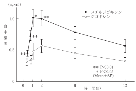
図 メチルジゴキシンの単回投与後のメチルジゴキシンの血中濃度
