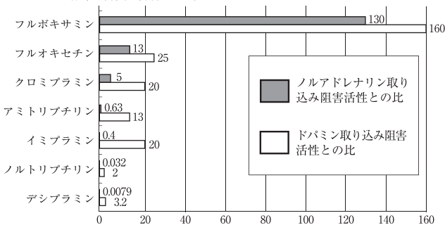
図1 セロトニンとノルアドレナリン及びドパミンの相対的取り込み阻害活性 (注)デシプラミンは販売中止品、フルオキセチンは国内未発売品
