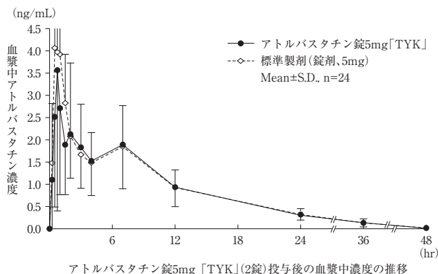
アトルバスタチン錠5mg「TYK」(2錠)投与後の血漿中濃度の推移
