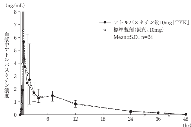
アトルバスタチン錠10mg「TYK」(1錠)投与後の血漿中濃度の推移
